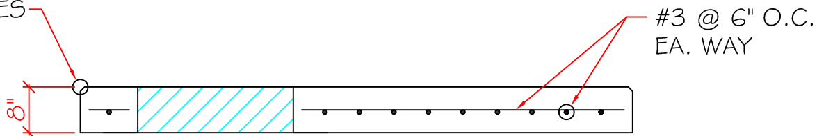
ELEVATION
